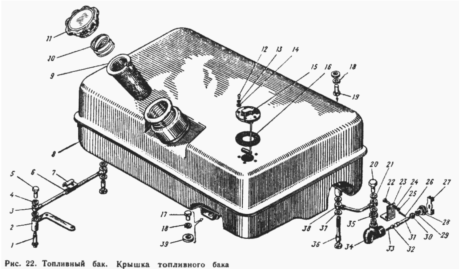
Рис. 22. Топливный бак. Крышка топливного бака.
